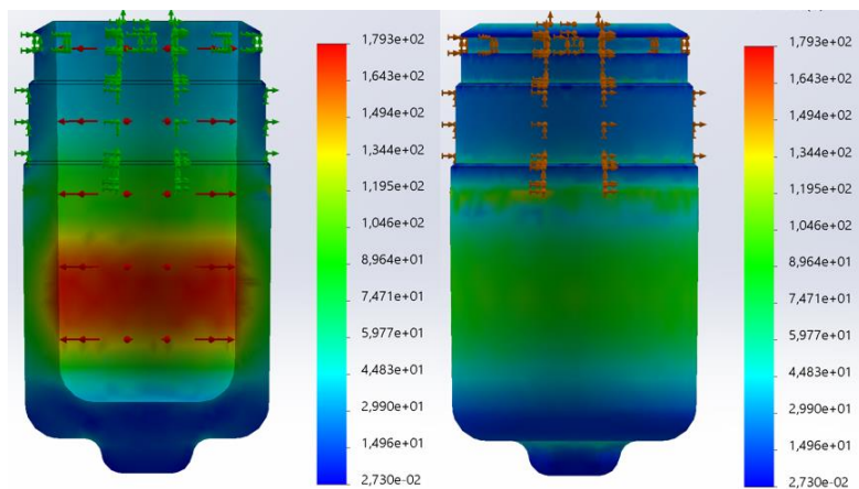
Şekil 6. 40 lt/dk filtre muhafazası iç çapta 2mm inceltmiş (ikinci tasarım).
