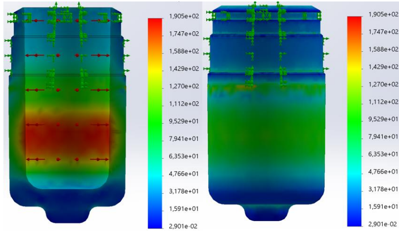
Şekil 8. 40 lt/dk filtre muhafazası iç çapta 3 mm inceltilmiş (üçüncü tasarım).
